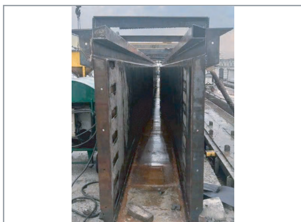
■ Dầm I33M căng sau
